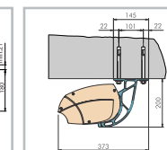
Deckenmontage M&F Kasette 2000
