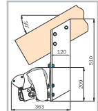
Dachsparrenmontage M&F Hülse 2000
