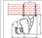
Deckenmontage M&F Hülse 2000
