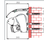
Wandmontage M&F Hülse 2000
