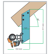
Dachsparrenmontage
