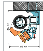
Deckenmontage
